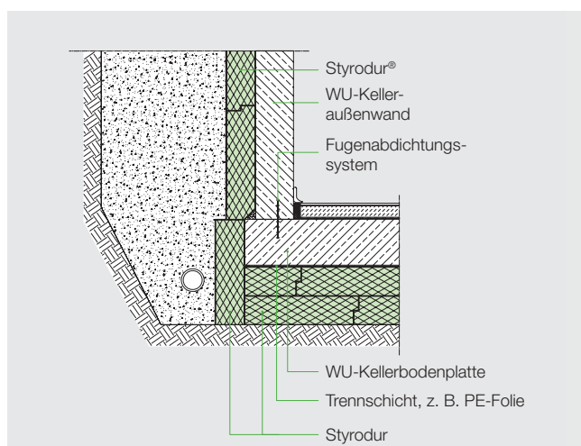
Abb. 18b: Anschluss gedämmte Bodenplatte an aufgehende Kelleraußenwand mit Styrodur Hybrid
