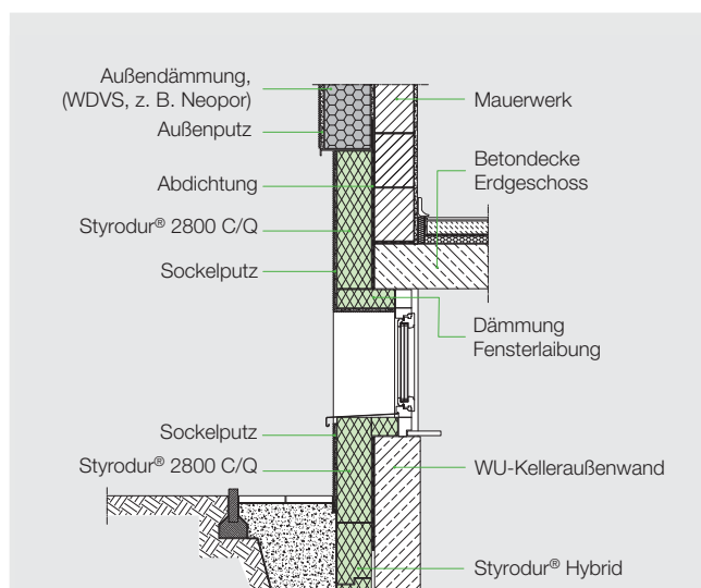
Abb. 19: Wärmebrückenfreie Dämmung im Fensterbereich.
