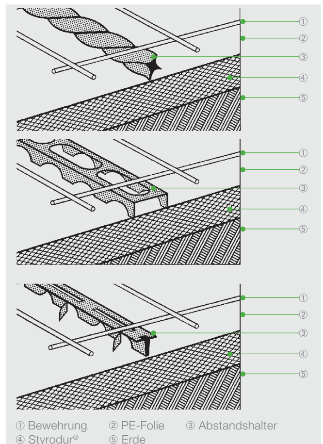
Abb. 10: Begehbare Kunststoffabstandshalter für die waagerechte Bewehrung. Durch die Profilhöhe ist die Betonüberdeckungshöhe vorgegeben.
