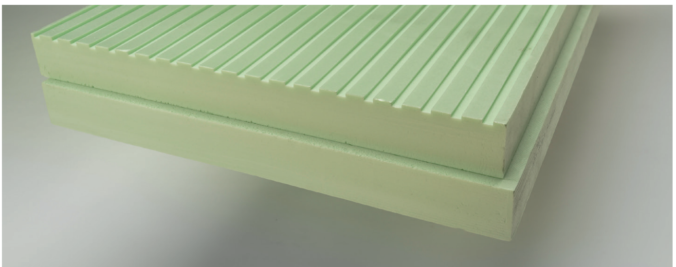
Abb. 32: Styrodur® Hybrid-Platte mit Längsrillen auf einer Oberflächenseite und umlaufendem Stufenfalz
