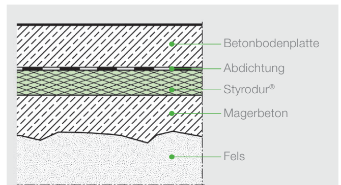
Abb. 7: Ausgleichsschicht aus Magerbeton bei Baugrund Fels.
