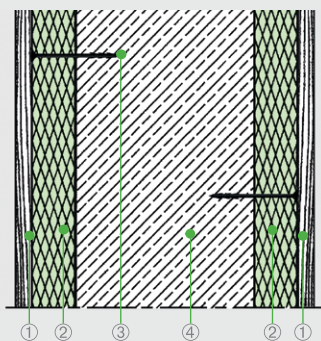
Abb. 26: Einstellen in die Schalung und Befestigen der Styrodur 3035 CS-Platten mit Kunststofferdnägeln.
