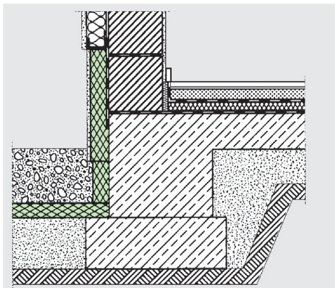
Abb. 12: Möglichkeiten der Fundamentdämmung gegen Unterfrieren.
