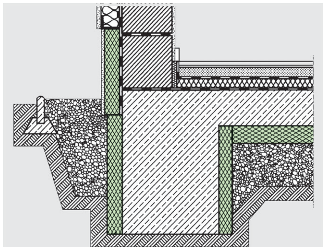
Abb. 11: Fundamentdämmung und Anschluss an das außenliegende Wärmedämmverbundsystem.
