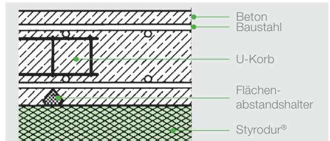
Abb. 9: Begehbarer Flächenabstandshalter aus Faserbeton für die untere Bewehrung und Baustahlgewebeunterstützungskorb für die obere Bewehrung der Bodenplatte.
