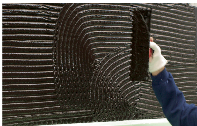
Abb. 16: Vollflächiges Verkleben der Dämmplatten bei drückendem Wasser.
