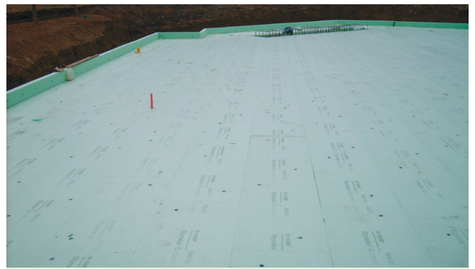
Abb. 40: Für eine exakte und wärmebrückenfreie Bodenplatte sind zwei wesentliche Faktoren maßgebend: die bauaufsichtlich zugelassene, dreilagige Dämmschicht aus Styrodur sowie eine professionelle Arbeitsvorbereitung mit verständlichen Montage- und Verlegeplänen.
