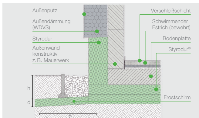
Abb. 14: Hinweis zur Ausführung eines Frostschirms.
