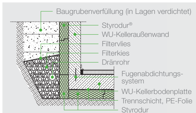
Abb. 18a: Fußpunkt der Perimeterdämmung. Die Styrodur-Platte steht auf dem Fundament auf.
