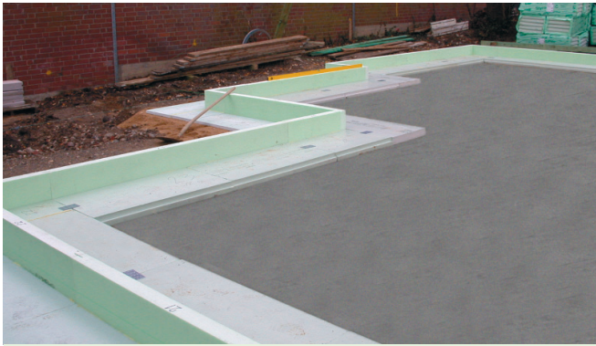
Abb. 37: Um in Teilbereichen eine kostenintensive Gründung bis zur Frosttiefe zu vermeiden, ist ein Frostschild nach EN ISO 13793 erforderlich. Dieser wird werkseitig an das Randelement angebracht und als waagrechte Erdreichdämmung eingesetzt.
